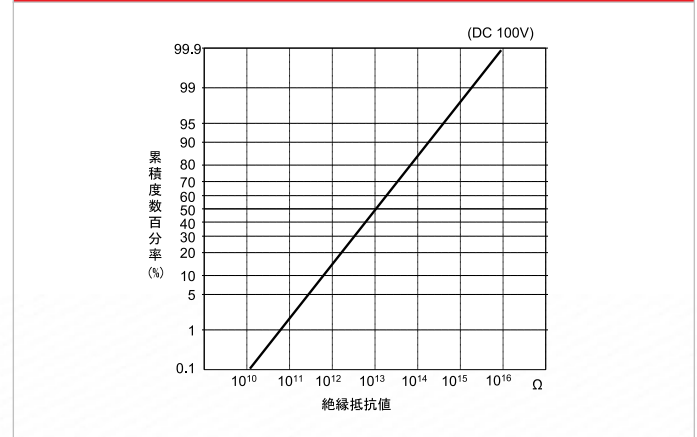
絶縁抵抗値
