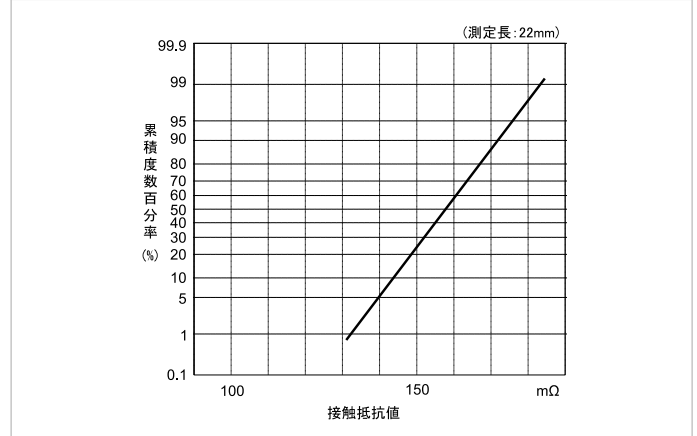
接触抵抗値
